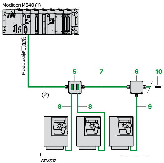
通过分管管连接的Modbus串行连接架构示例
