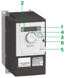
ATV312H075M2，前面板上的门关闭，有保护盖5：STOP/RESET 和 RUN按钮可用
