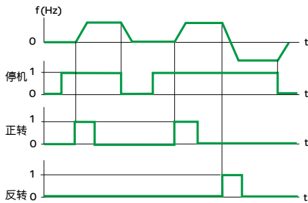
3线控制运行示例
