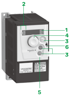
ATV312H075M2前面板上的门关闭，无保护盖5：STOP/RESET 和 RUN按钮可用
