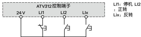
3线控制接线图
