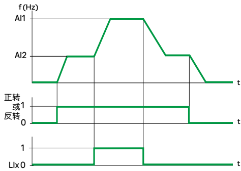
给定值切换示例
