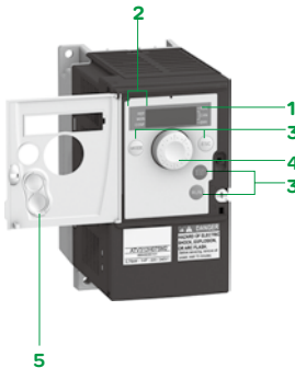
ATV312H075M2，前面板上的门打开
