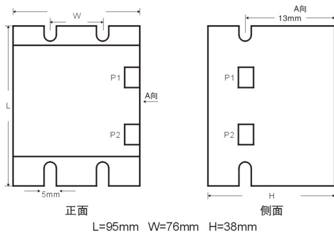
安装图纸（正面、侧面）
